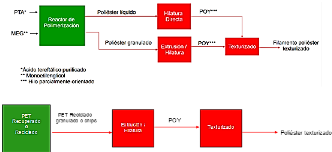
Diagrama del proceso productivo de PFTT
